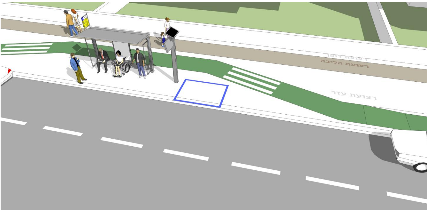
תרשים 5.37 מפגש שביל אופניים עם תחנת אוטובוס ללא מפרץ
